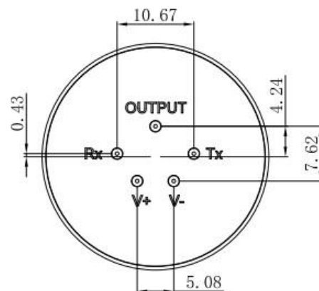
仰视图
